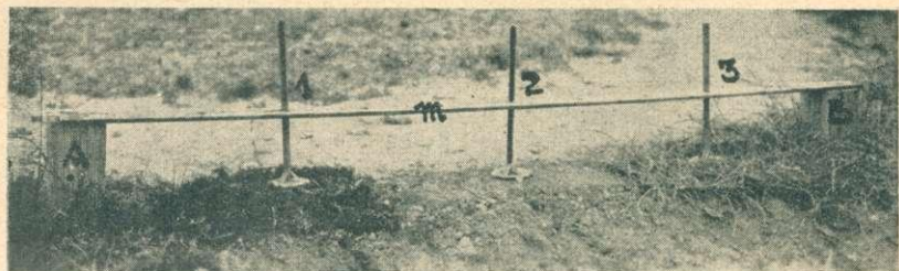
1. kép. Talajfelfagyásmérő.
