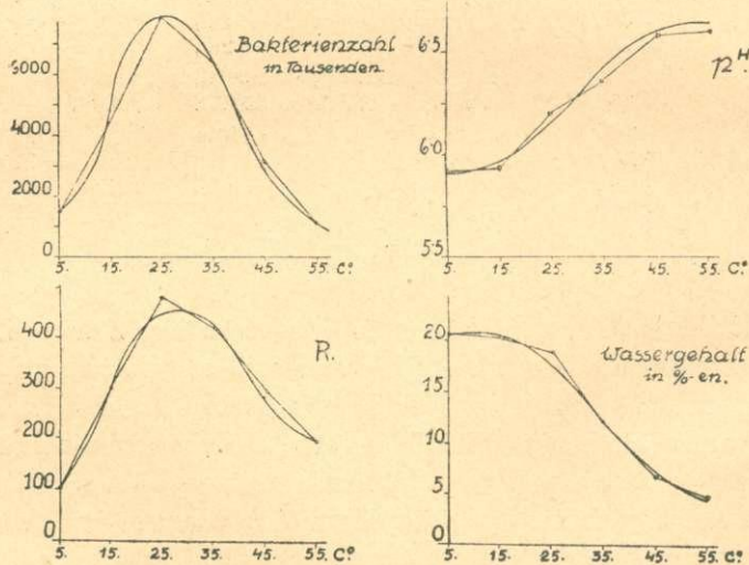
13. kép. A talaj baktériumszámának, az R-tényezőknek, a ph-értékeknek és a talaj víztartalmának változásai a 2. sz. kísérlet alapján.
