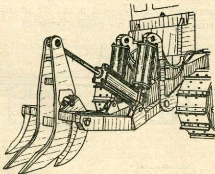
4. ábra. K2A hidraulikus tuskókiemelő gép
