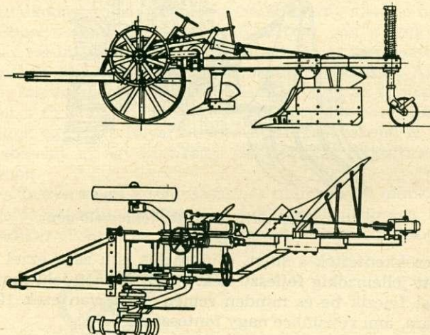
5. ábra. PP—50 mélyforgató eke
