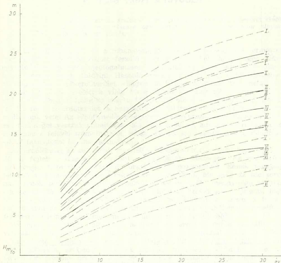
3. ábra. Közönséges akácok és akácfajták főállományának átlagos magassága, fatermési osztályonként a különböző fatermési táblák alapján (pont-vesszős vonal Fekete Z. 1960, szaggatott vonal Sopp L. 1974; folytonos vonal akácfajták Gödöllő 1984)
