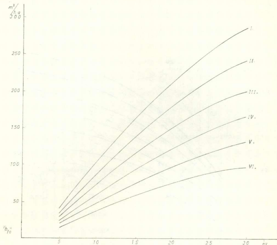
4. ábra. Akácfaajták főállományának földfeletti bruttó összes fatérfogata fatermési osztályonként
