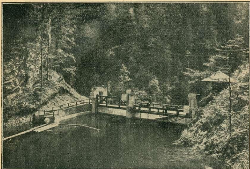
4. kép. A Rasthöhe-i gát telt medence mellett. Jobbról balra látható a tulajdonképpeni gát, az árapasztó, majd a balszélén az úsztatócsatorna kiágazása. (Passer felv.)
