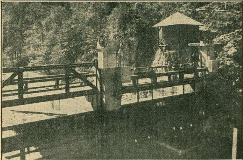
5. kép. Ugyanaz. Jól láthatók a gátat záró emelő, az árapasztót záró süllyeszthető kapu állítását megkönnyítő betonellensúlyok, valamint a zúgókapuk emelőszerkezete. (Passer felv.)
