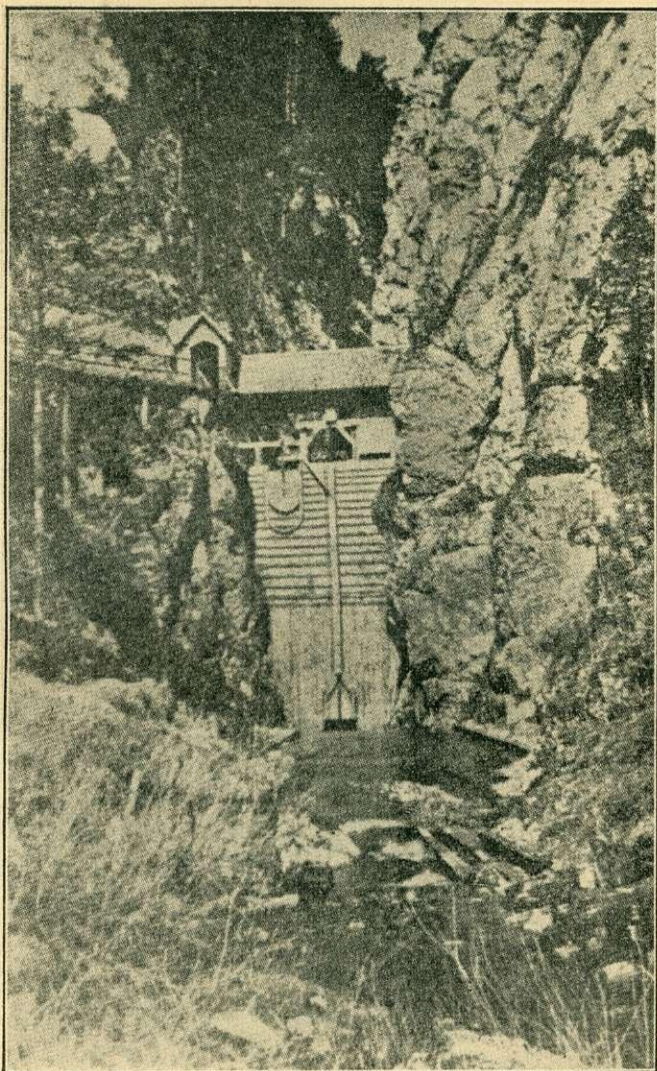
1. kép. A Taschl-Graben vízgyűjtője üres gátmedence mellett, a vízfal felől nézve. (Kühne felv.)
