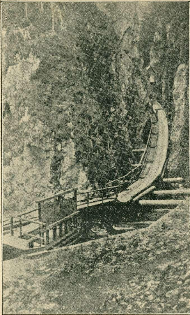
2. kép. A Taschl-Graben-i gátból kiinduló vizes csúsztató a sebességcsökkentő medencével, háttérben kissé látszik a gát is. (Kühne felv.)
