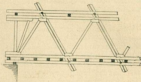
23. sz. ábra. Ibianski-féle rácestartó.
