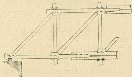
21. sz. ábra. Rybter-féle rácstartó.
