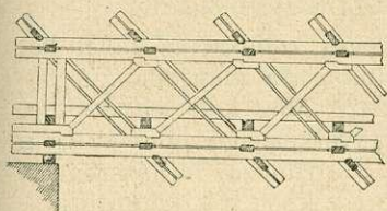
22. sz. ábra. Pintorski-féle rácestartó.
