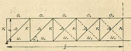
25. sz. ábra. A Howe- és Rychter-féle hídtartó- szerkezetek mintája.
