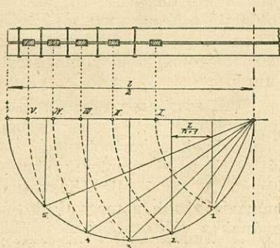
12. sz. ábra. Ékkiosztás szerkesztés útján
