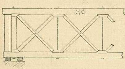
20. sz. ábra. Howe-féle rácstartó.
