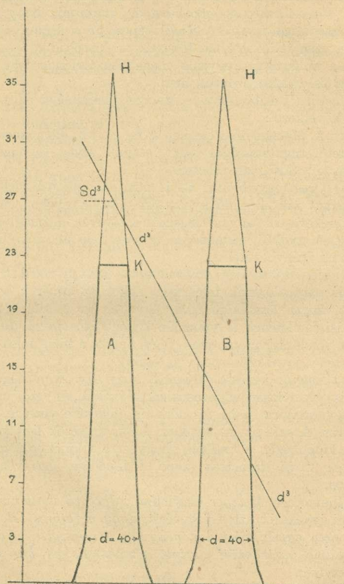
2. sz. ábra. Jaccard munkájának 2. ábrája után. — B Egy valódi Picea-törzs alakrajza. A Egy Metzger elmélete alapján mint egyenlő ellenállású Piceatörzs rajza. Jelmagyarázat, mint az első ábrán.
