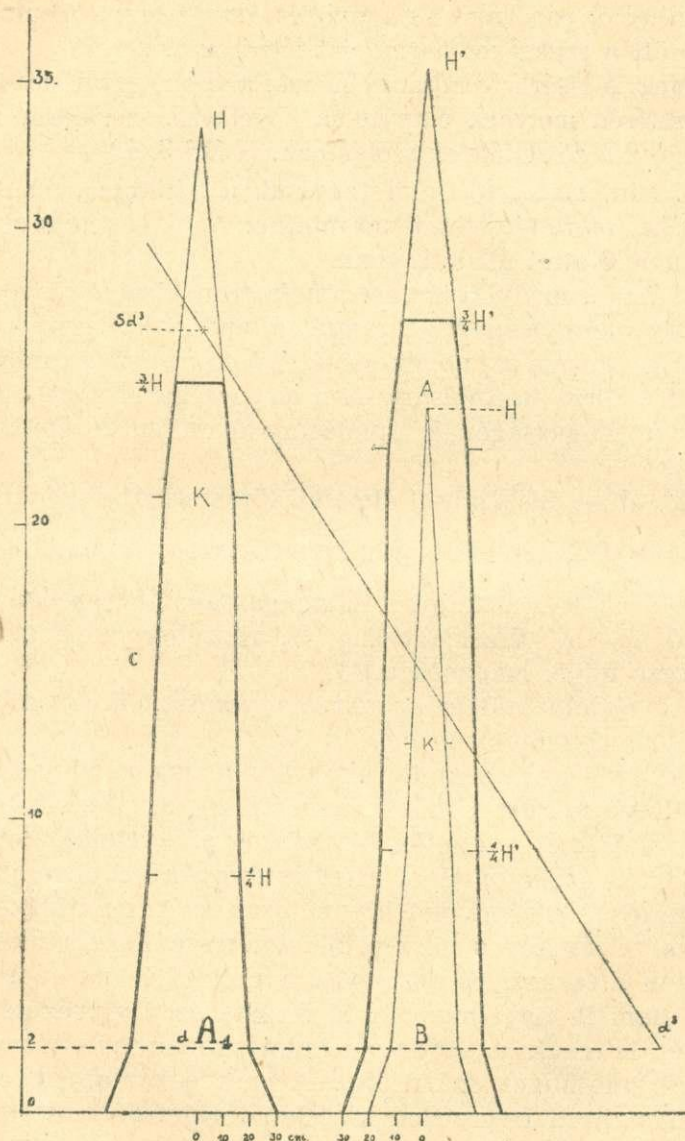
3. sz. ábra. Jaccard munkájának 5. sz. rajza után. — A Egy a vízvezető elmélet alapján szerkesztett elméleti forma, n = \frac{d_{3/4}h}{d_{1/4}h} = 0.52 . — B Egy 50 éves valódi Picea-törzs n = 0.47 . — A1 Egy 74 éves valódi Piceatörzs (Winterthur) n = 0.57 . — A többi jelzés, mint az első ábránál.
