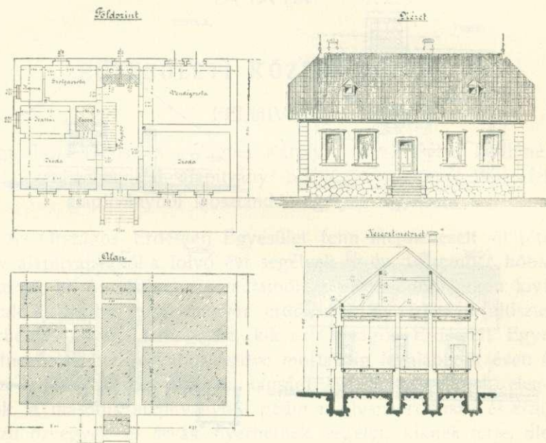
4. ábra. A šipovoi erdőgondnoksági irodaépület.
