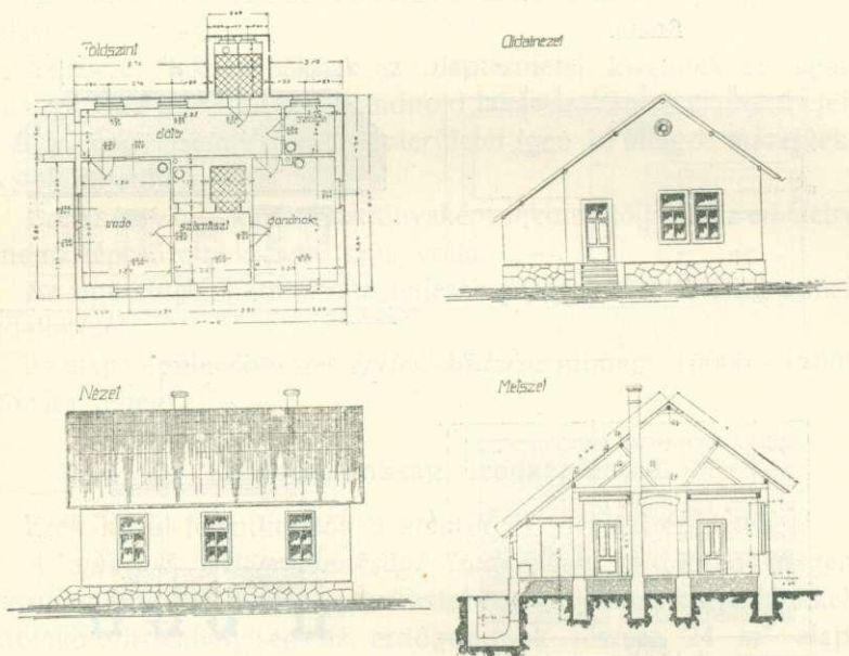
5. ábra. A nemilai irodaépület.
