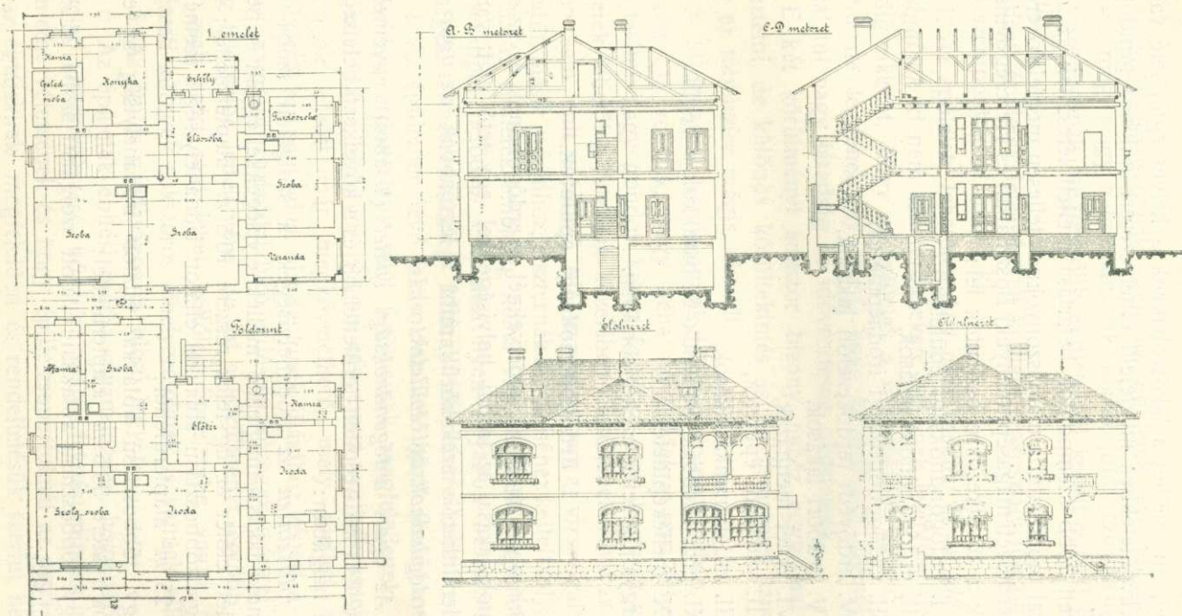
1. ábra. Az ugari erdőgondnoksági épület.
