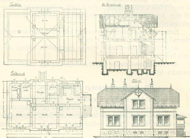
3. ábra. A Šipovoi erdőgondnoki lak.
