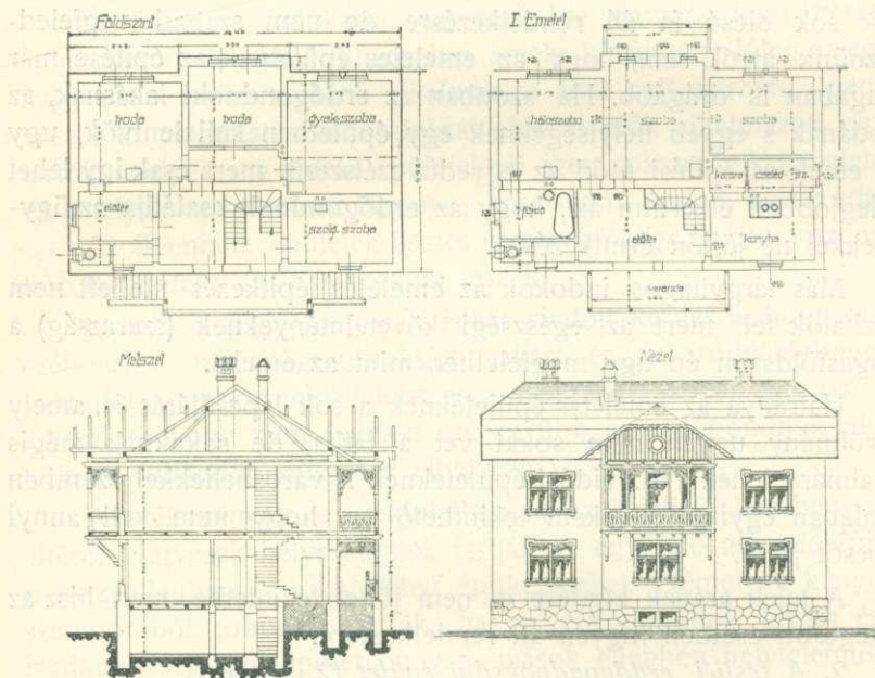
2. ábra. A teslići erdőgondnoksági épület.
