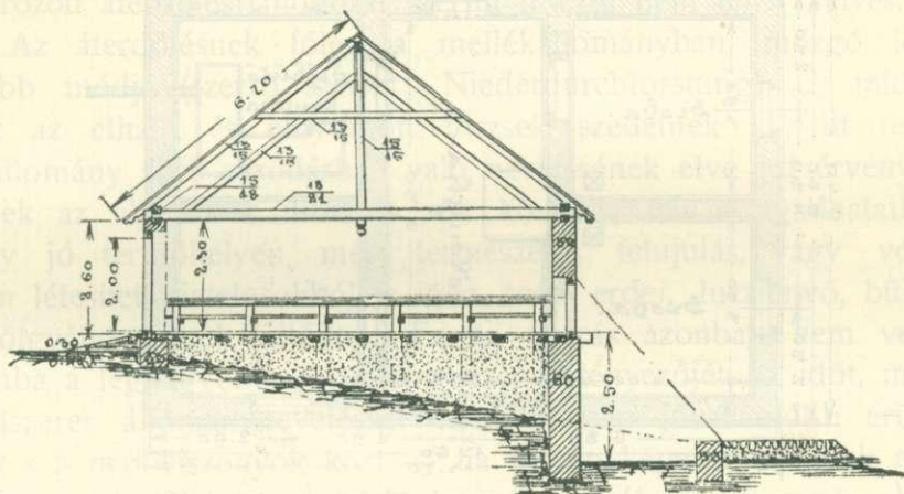
12. kép. Havasi istálló keresztmetszete.
