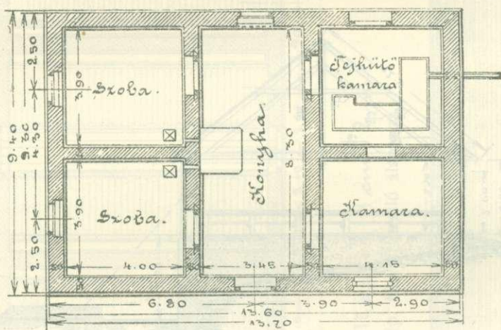
13. kép. Havasi majoroslak alaprajza.
