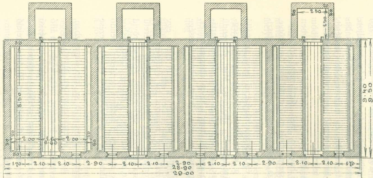
10. kép. Havasi istálló alaprajza.
