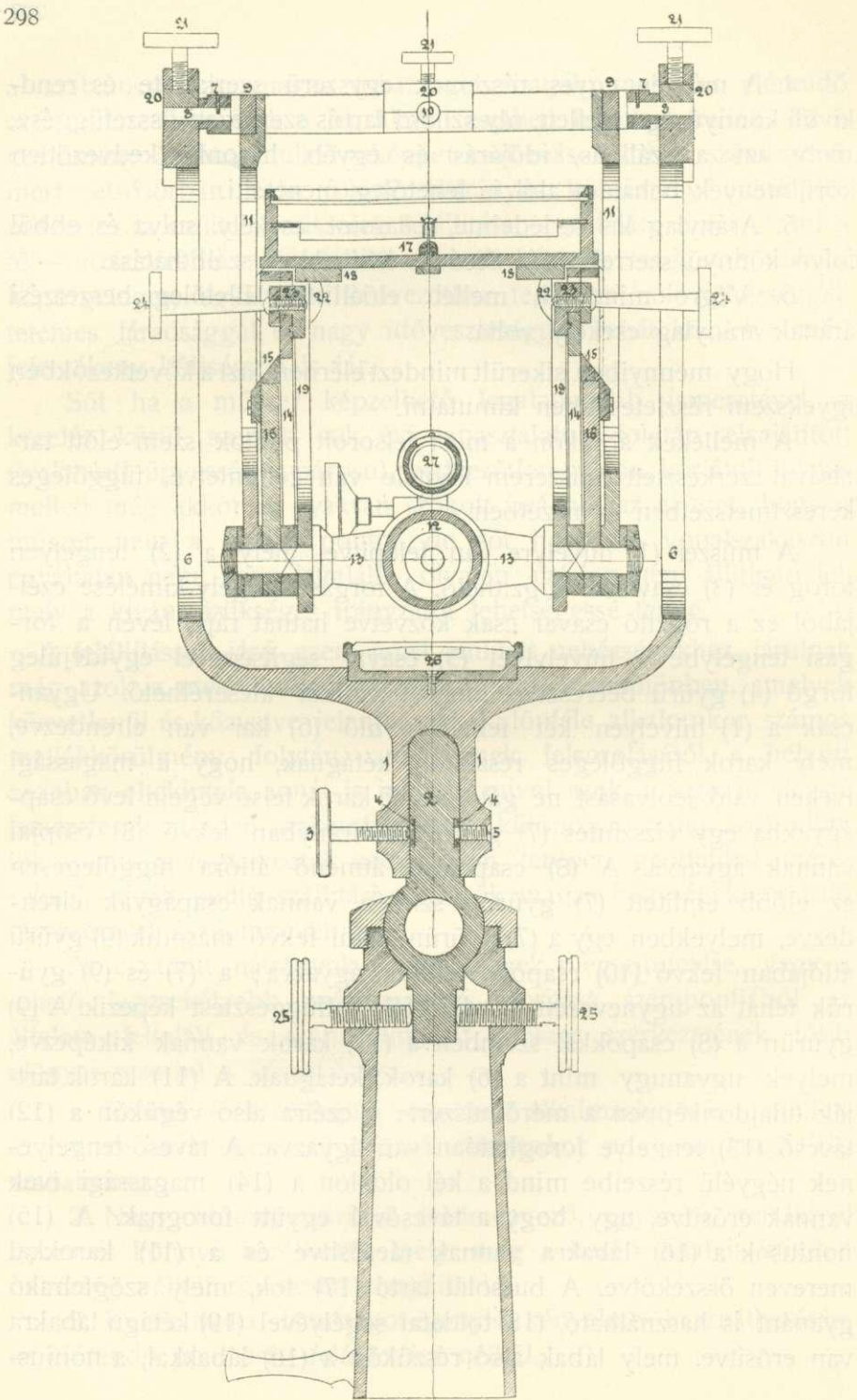
16. kép. Önműködően szintesre álló mérő műszer (metszet).
