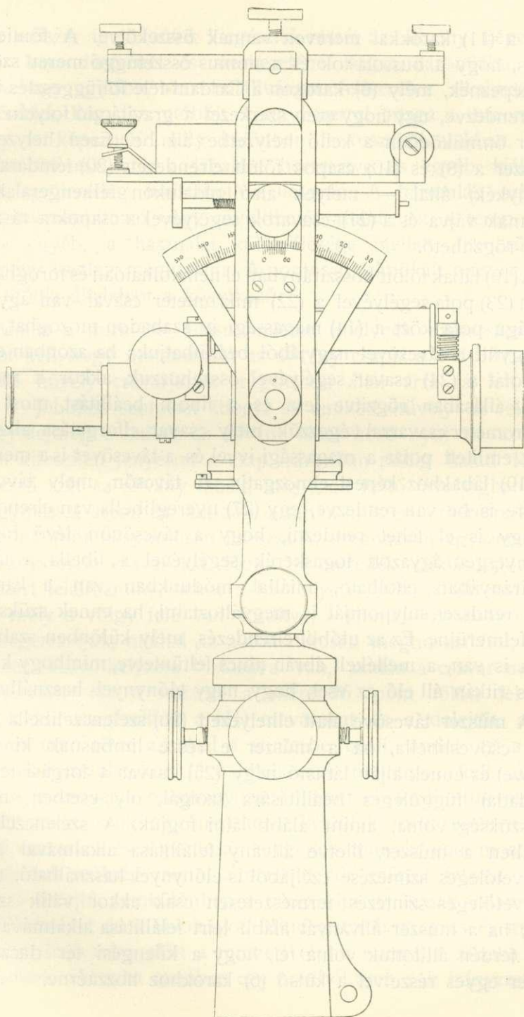
17. kép. Önműködően szintesre álló mérő műszer (oldalnézet).
