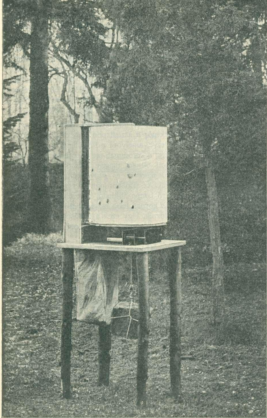
19. kép. Friedrich-féle lepkefogó működésben.
