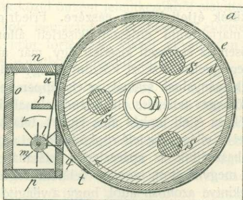
18. kép. Friedrich-féle lepkefogó szerkezete.
