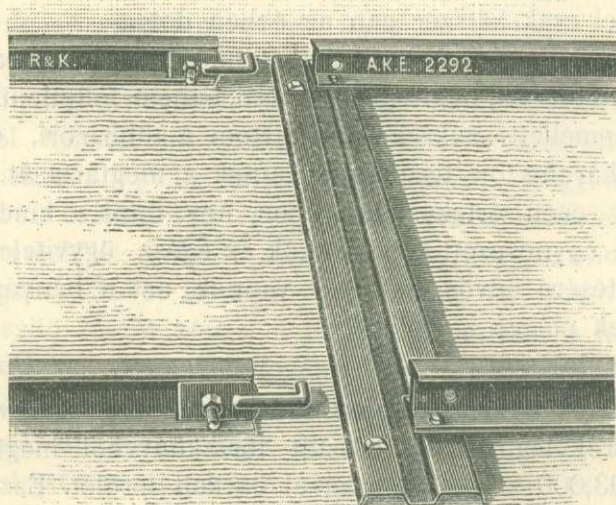
15. ábra. A vágány kapcsolat előtt (aczéltalpakon).
