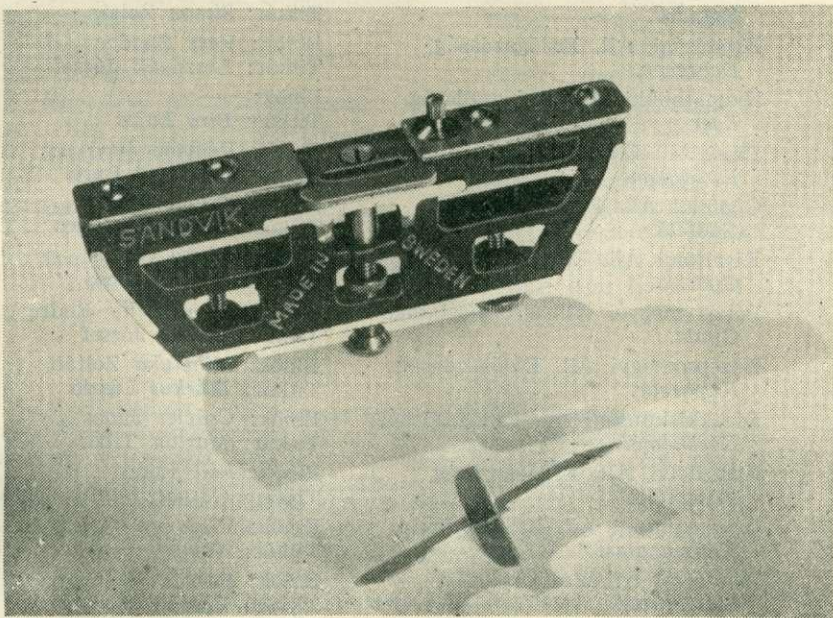
Gyalufog-rövidítő berendezés
